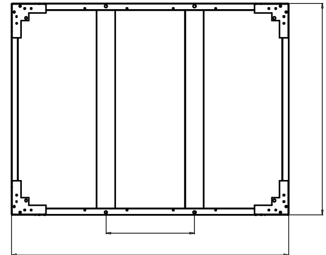
SEZ. A-A
